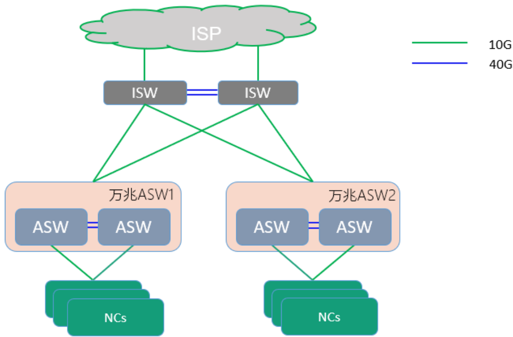
网络架构逻辑分区
